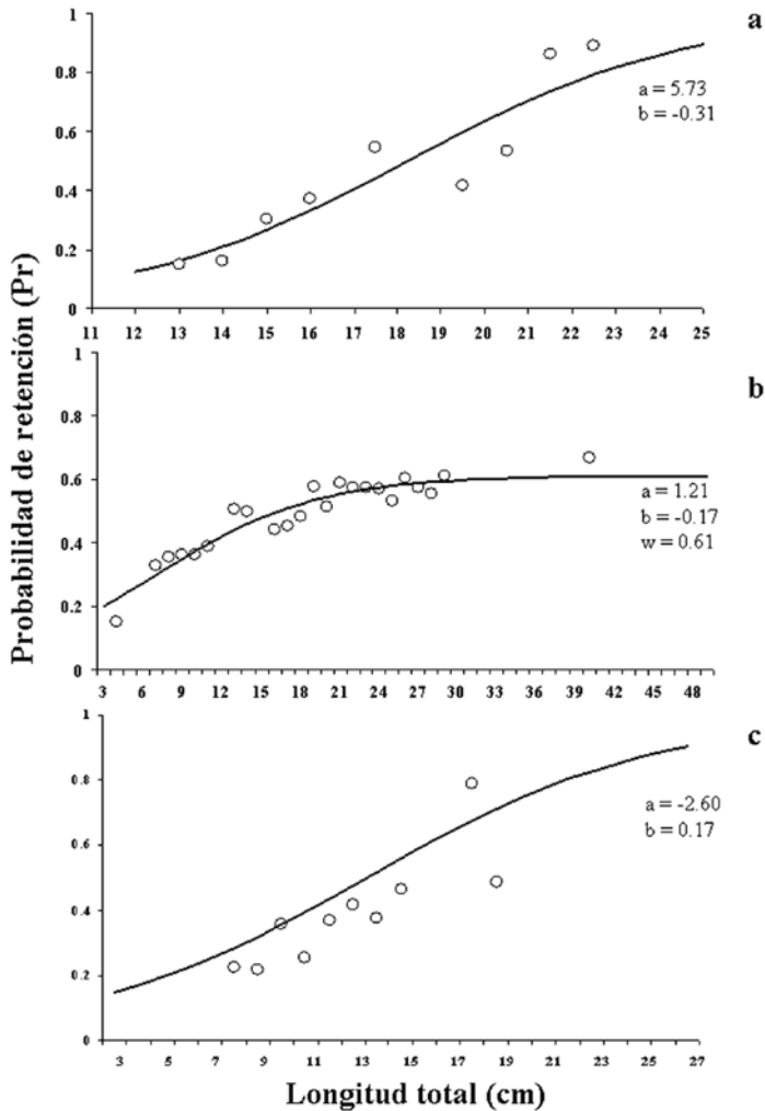
Figura 9. Curvas de selectividad de la red prototipo para: a) Litopenaeus occidentalis , b) familia Sciaenidae y c) familia Engraulidae. En cada caso se muestran los parámetros significativos estimados.
