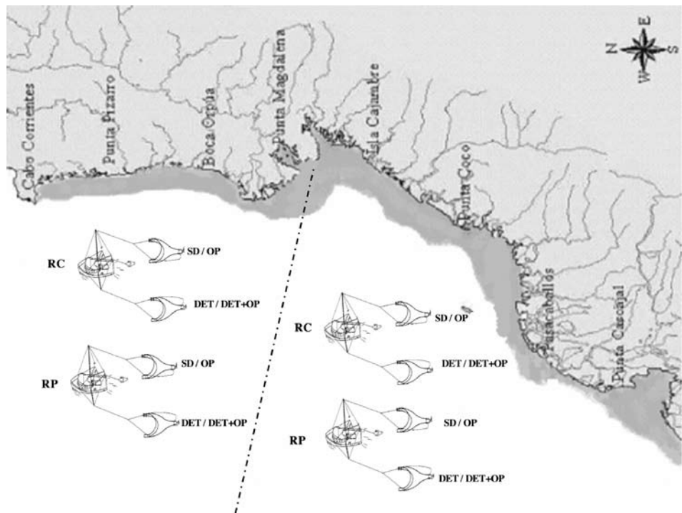
Figura 2. Esquema del diseño de pesca experimental donde los factores subárea, tipo de red y presencia de dispositivo, son cubiertos con la operación simultánea de dos embarcaciones de la flota industrial de arrastre del Pacífico, RC: red convencional, RP: red prototipo, DET: dispositivo excluidor de tortugas, SD: red sin dispositivo.
