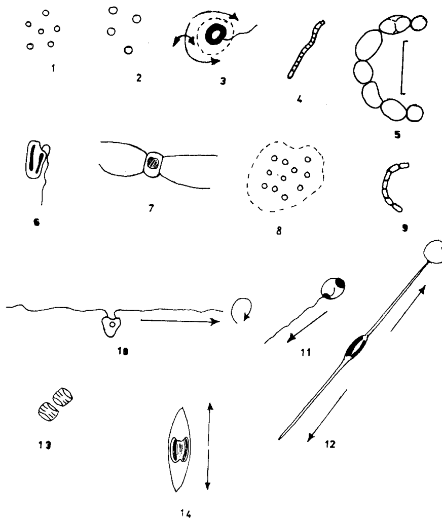
Figura 2. Iconos correspondientes a las formas de fitoplancton listadas en la tabla 6. Las flechas indican la dirección del movimiento observado. La escala en el icono 5 equivale a 10 \mu m.
