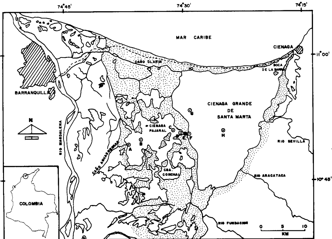
Figura 1. Area de Estudio. A = Boca Caño Aguas Negras; B = El Morro; C = Buenavista (zona occidental); D = Boca Caño Grande en Cga. de Pajalar; E = Caño Grande; F = Boca Caño Grande en CGSM; G = CGSM, al norte de Caño Grande; H = Centro de la CGSM.
