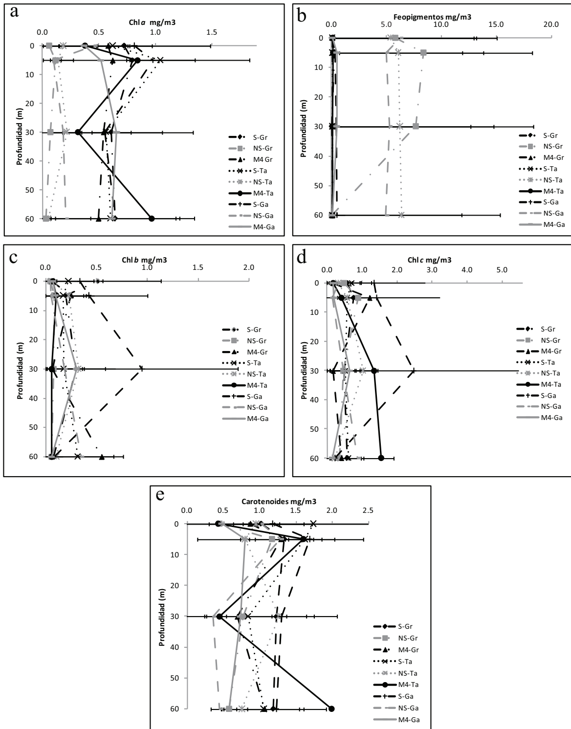
Figura 5. Perfiles de clorofila a y pigmentos accesorios para los seis muestreos correspondientes a períodos de surgencia y no surgencia en las estaciones Gaira (Ga), Taganga (Ta) y Granate (Gr) a 0, 5, 30 y 60 m de profundidad. (a) Clorofila a . (b) Feopigmento a . (c) Clorofila b . (d) Clorofila c . (e) Carotenoides. M4: Muestreo 4. S: surgencia. NS: no surgencia.
