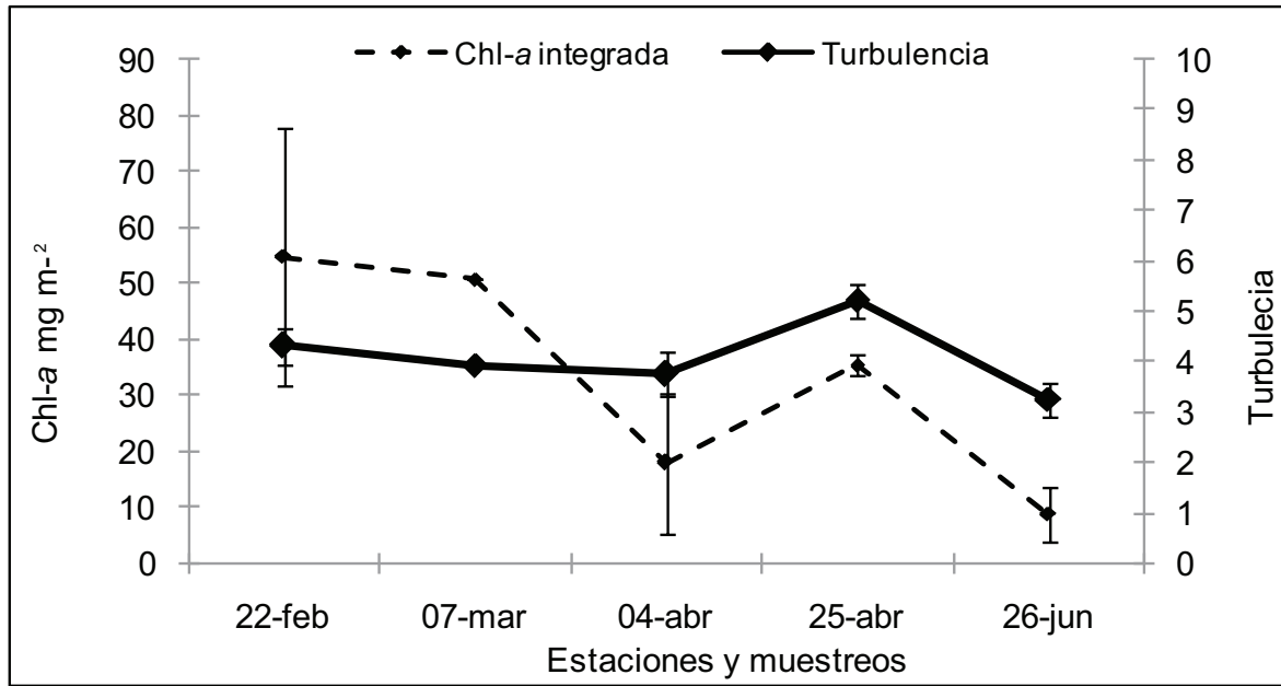
Figura 6. Variación de la concentración de clorofila a integrada en la columna de agua (0-60 m) y su relación con la turbulencia del agua en el período febrero–junio de 2008 para las ensenadas de Gaira (Ga) y Granate (Gr) y la bahía de Taganga (Ta).
