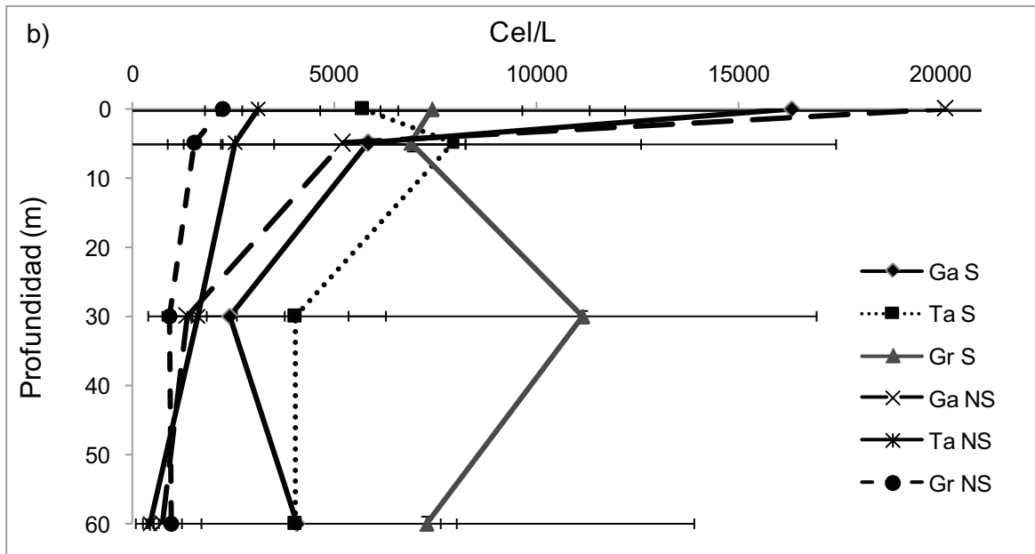
Figura 3. Densidad celular fitoplanctónica (cel/L) registrada para las estaciones Gaira (Ga), Taganga (Ta) y Granate (Gr) conforme a seis muestreos bajo condiciones de surgencia (S) y no surgencia (NS). (a) Densidades totales para la columna de agua de 0 a 60 m de profundidad. (b) Densidades totales promedio propias de las profundidades 0, 5, 30 y 60 m del agua.
