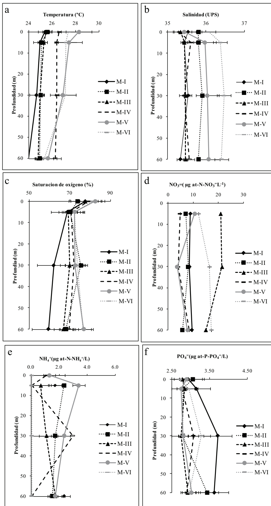
Figura 2. Perfiles de (a) temperatura, (b) salinidad, (c) porcentaje de saturación de oxígeno, (d) concentración de NO 3 - , (e) concentración de NH 4 + y (f) concentración de HPO 4 - en la columna de agua, para la totalidad de los muestreos a 0, 5, 30 y 60 m de profundidad. M-I: muestreo 1, M-II: muestreo 2, M-III: muestreo 3, M-IV: muestreo 4, M-V: muestreo 5, M-VI: muestreo 6.
