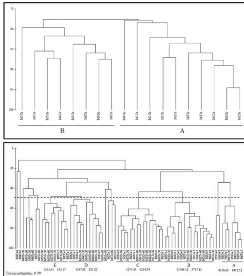
Figura 4. Análisis de clasificación cualitativo de presencia/ausencia (a) y cuantitativo de Bray-Curtis (b) para la comunidad fitoplanctónica de la zona costera del departamento del Magdalena, bajo condiciones de surgencia y no surgencia usando como técnica de ligamiento el método UPGMA. M1, 2, ..., 6: muestreo uno, dos, ..., seis. Gr: Estación Granate. Ta: Estación Taganga. Ga: Estación Gaira. A, B, C...: indican agrupaciones formadas, como las densidades celulares promedio de cada grupo en cel/L.
